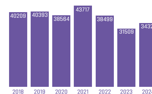
Evolution des tonnages de végétaux valorisés
