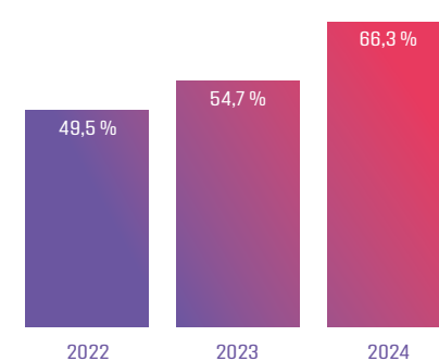
Taux de valorisation des déchets non dangereux, non inertes de la Dordogne
