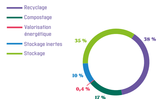
Taux de valorisation des déchets de Dordogne en 2024
