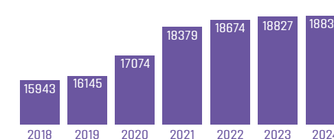
Evolution des tonnages de verre valorisés
