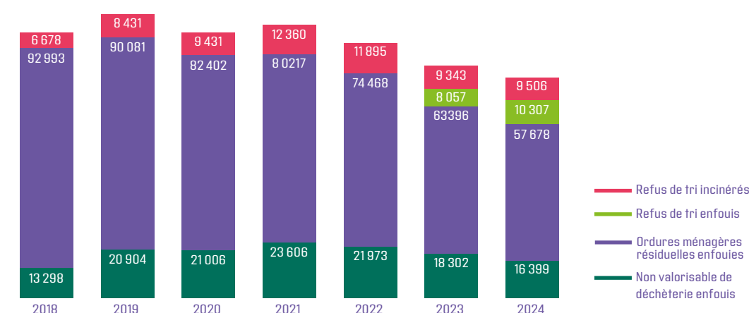
Évolution des tonnages de déchets ménagers résiduels
