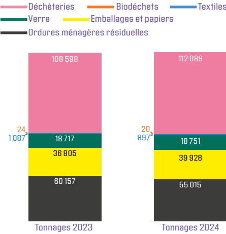
Évolution des tonnages collectés
